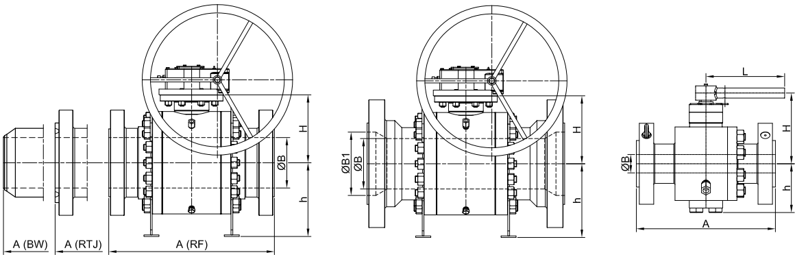
ASME CLASS 150
