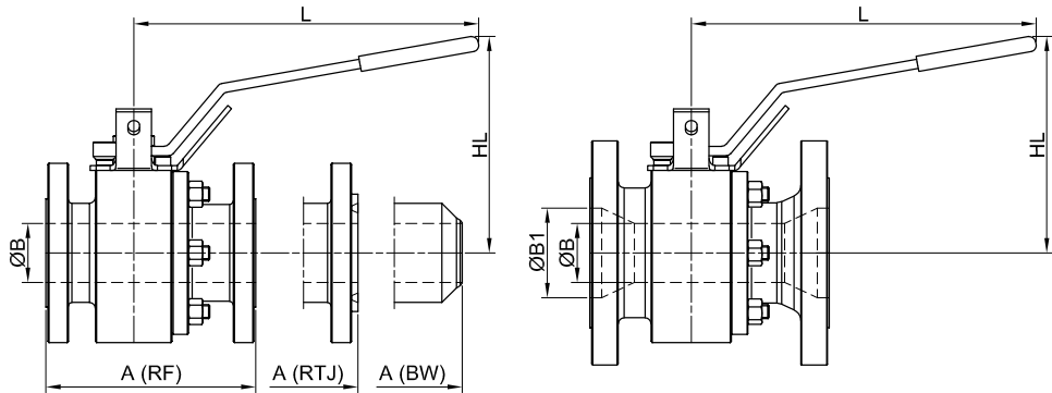
ASME CLASS 150
